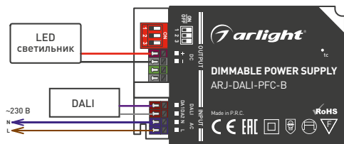
Рисунок 1. Подключение источника напряжения при использовании интерфейса DALI
