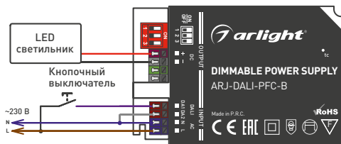
Рисунок 2. Подключение источника напряжения при управлении кнопкой (Push Dim)
